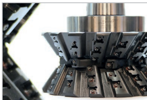
Special mills Fresas especiales
